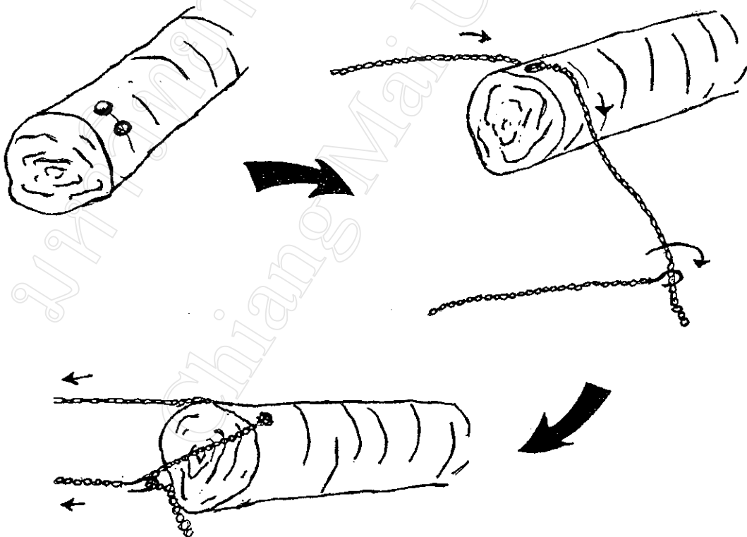
ภาพที่ 58 การร้อยโซ่เข้ากับซุง
