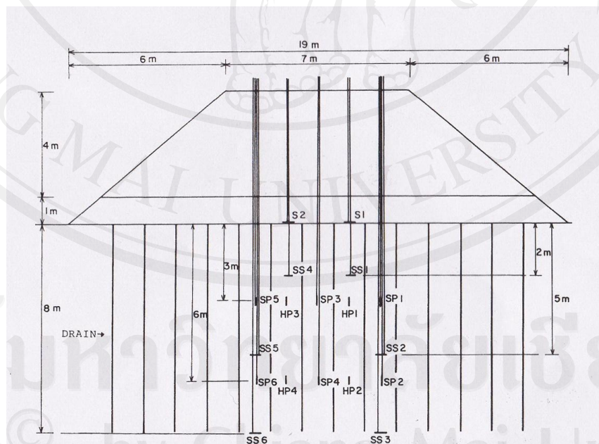
รูป 1.5 การติดตั้งเครื่องมือทดสอบ ที่มา: Bergado (1991)
