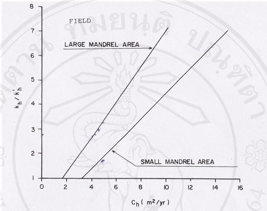
รูป 1.7 แสดงการคำนวณกลับค่าสัมประสิทธิ์การอัดตัวระบายน้ำในแนวราบ ( C_h ) ที่มา: Bergado (1991)
