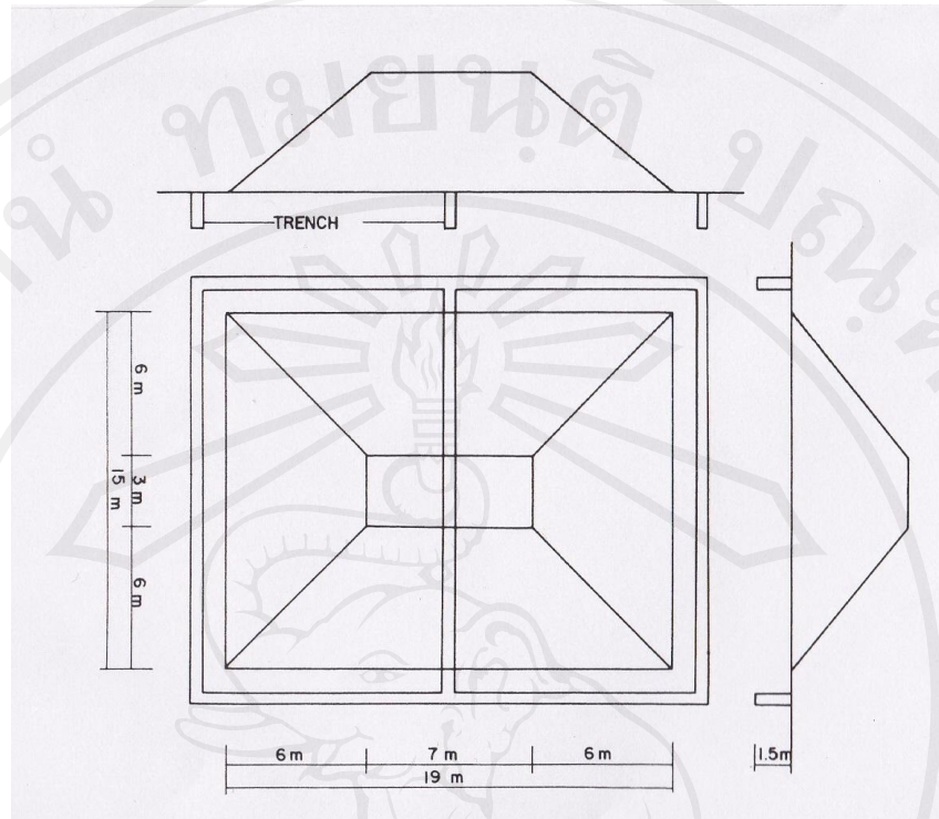
รูป 1.4 แผนและรูปตัดแสดงขนาดของดินถม (น้ำหนักรรทุก) ที่มา: Bergado (1991)
