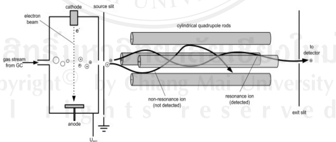
รูป 1.8 การเกิดไอออนของสารด้วยการใช้ EI เกิดเป็นอนุภาคมีประจุแล้วถูกผลักหรือดึงดูดเข้าสู่ส่วนแยกมวลควอดรูโพล (Quadrupole) (Agilent technologies, 2005)
