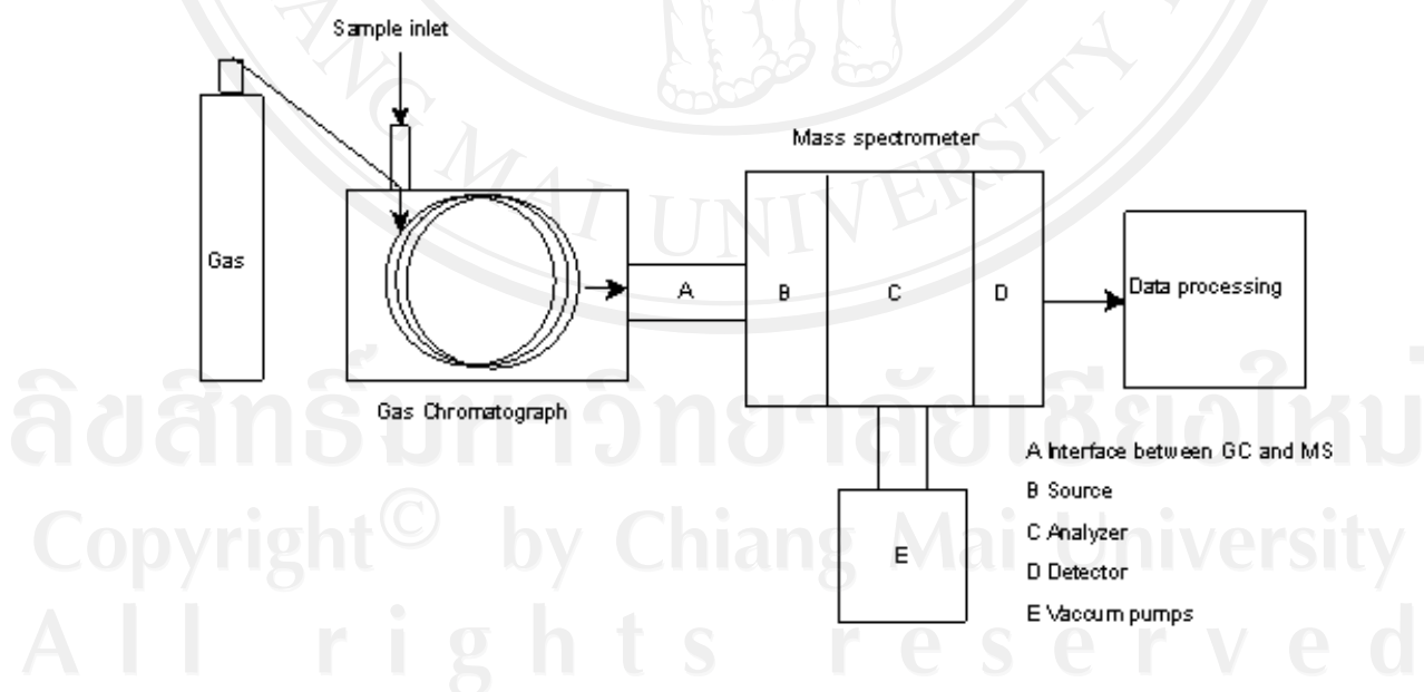
รูป 1.7 ระบบของแก๊สโครมาโทกราฟี-แมสสเปกโตรมิเตอร์ (พรเทพ, 2548)
