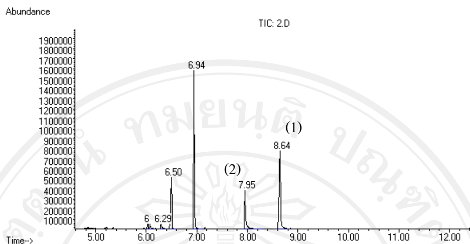
รูป 3.10 โครมาโทแกรมแบบ TIC ของวิธีการเก็บข้อมูลแบบ SIM ของแอมเฟตามีน เมทแอมเฟตามีน และ MA-d5 ที่เตรียมอนุพันธ์ด้วย HFBCl จากสารละลายมาตรฐานผสมแอมเฟตามีน เมทแอมเฟตามีน และ MA-d5 ความเข้มข้น 20 ไมโครกรัมต่อมิลลิลิตร
