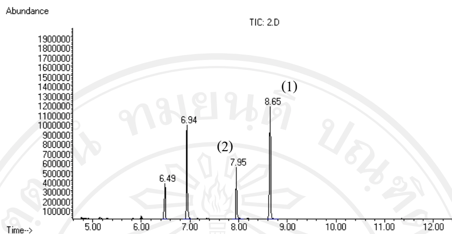
รูป 3.9 โครมาโทแกรมแบบ TIC ของวิธีการเก็บข้อมูลแบบ SIM ของแอมเฟตามีน เมทแอมเฟตามีน และ MA-d5 ที่เตรียมอนุพันธ์ด้วย HFBA จากสารละลายมาตรฐานผสมแอมเฟตามีน เมทแอมเฟตามีน และ MA-d5 ความเข้มข้น 20 ไมโครกรัมต่อมิลลิลิตร
