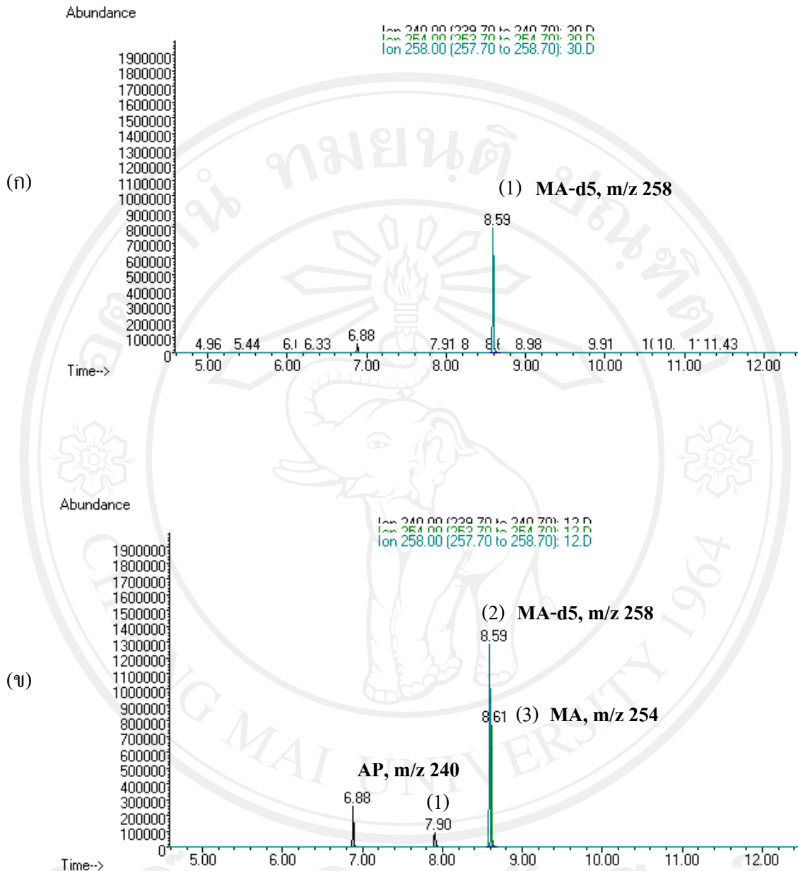
รูป 3.19 โครมาโทแกรมชนิด TIC ของวิธีการเก็บข้อมูลแบบ SIM ในเส้นผมของผู้เสพยาบ้า
