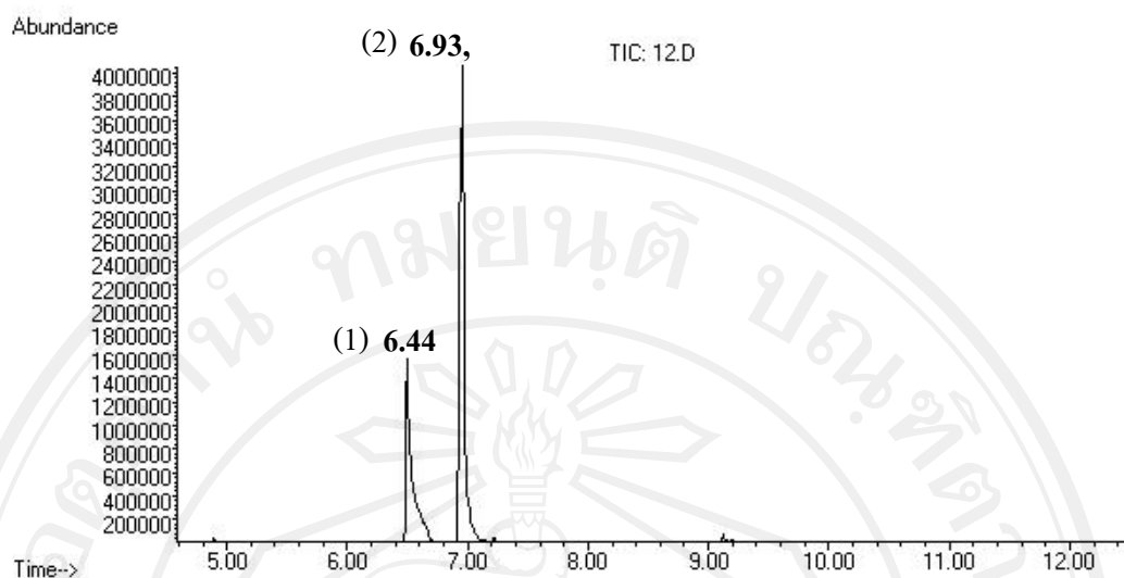
รูป 3.1 โครมาโทแกรมแบบเก็บไอออนทั้งหมด (Total chromatogram; TIC) ของวิธีการเก็บข้อมูลแบบ SIM ของแอมเฟตามีน เมทแอมเฟตามีน และ MA-d5 จากสารละลายมาตรฐานผสมแอมเฟตามีน ความเข้มข้น 4 ไมโครกรัมต่อมิลลิลิตร เมทแอมเฟตามีน และ MA-d5 ความเข้มข้น 1 ไมโครกรัมต่อมิลลิลิตร จากภาพ
