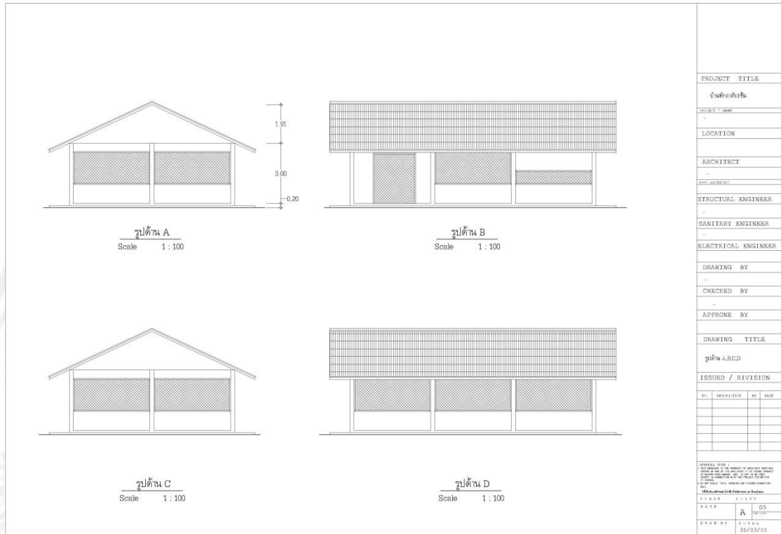
ภาพที่ ข 1 แปลนภายนอกอาคารโรงงานขนมจีน
