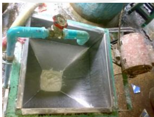
ภาพที่ ก 3 ลักษณะภายในเครื่องโรยแป้งขนมจีน
