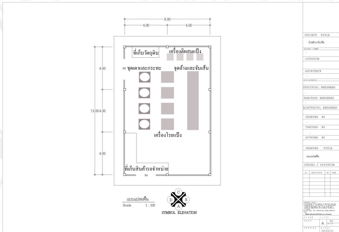
ภาพที่ ข 2 แปลนภายในอาคารโรงงานขนมจีน
