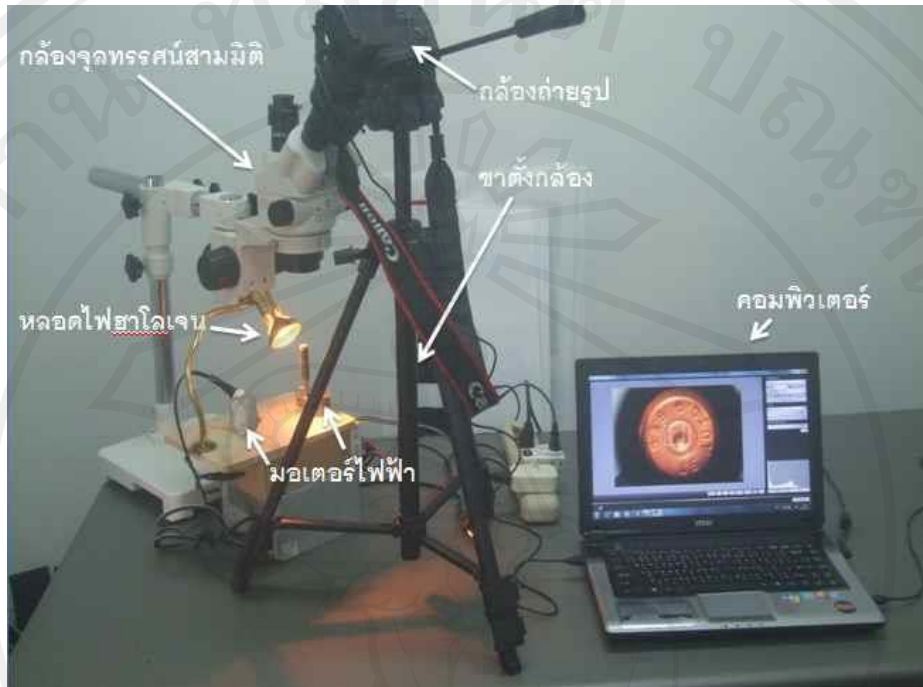
ภาพแสดงการจัดวางชุดอุปกรณ์
