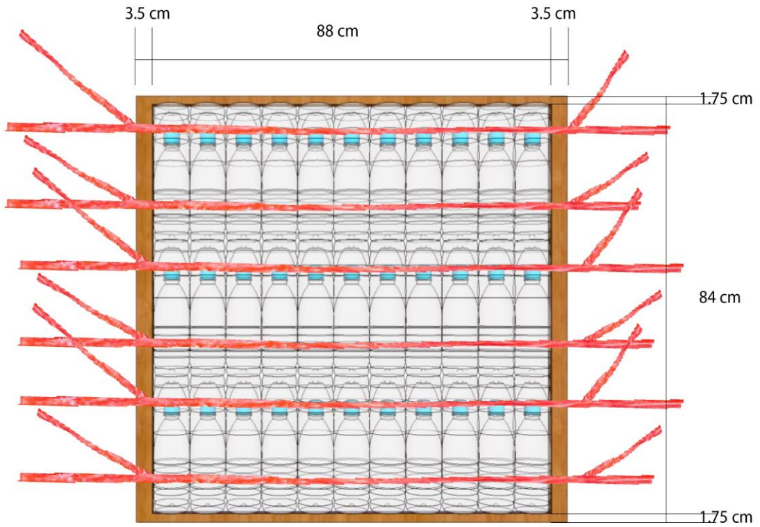
ชิ้นส่วนประกอบ แผงขวดน้ำดื่มพลาสติก ค้านข้างติดถนนส่วนกลาง
