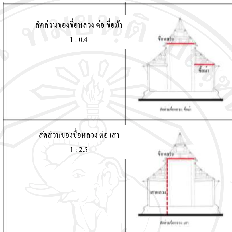
ภาพ 4-15 แสดงสัดส่วนวิหารล้านนาในจังหวัดเชียงใหม่ (ต่อ)
