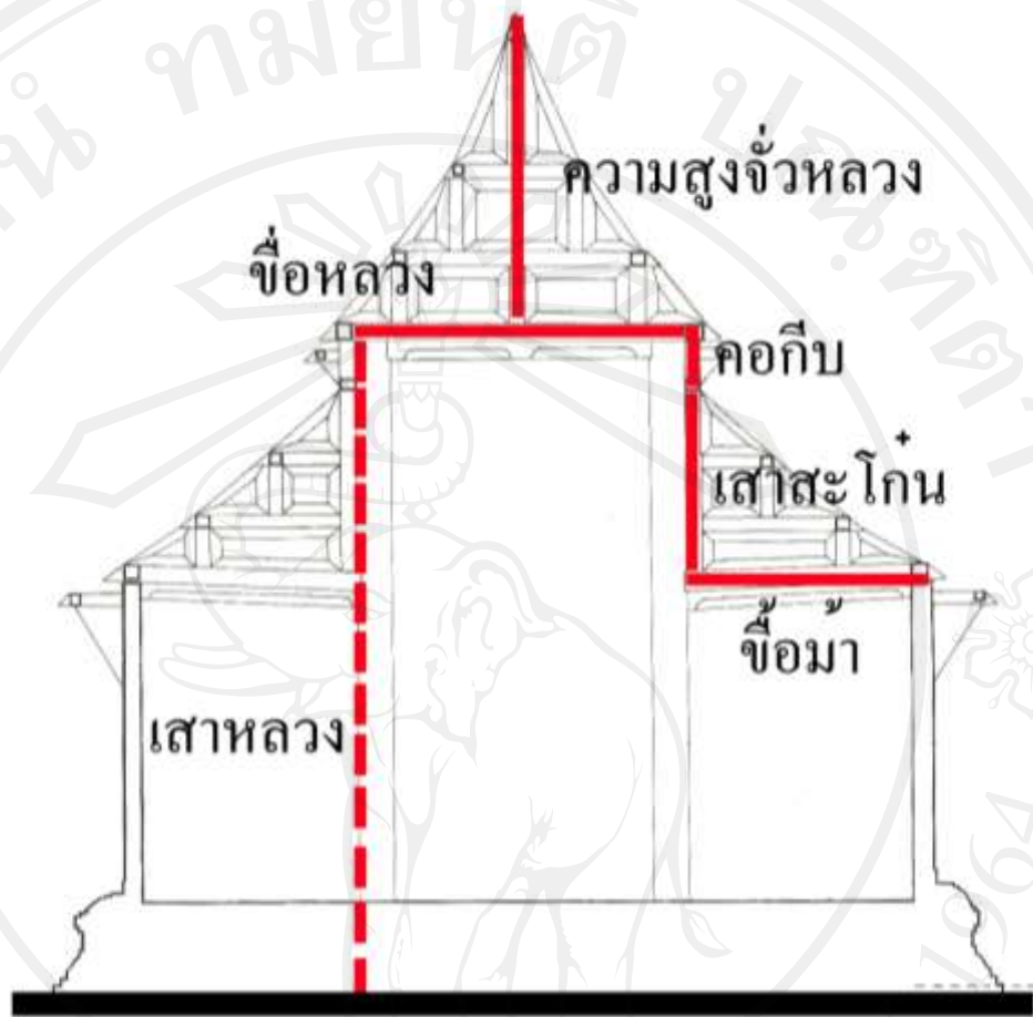
ภาพ 4-3 แสดงองค์ประกอบของโครงสร้างจั่วหลวงที่จะนำมาวิเคราะห์
