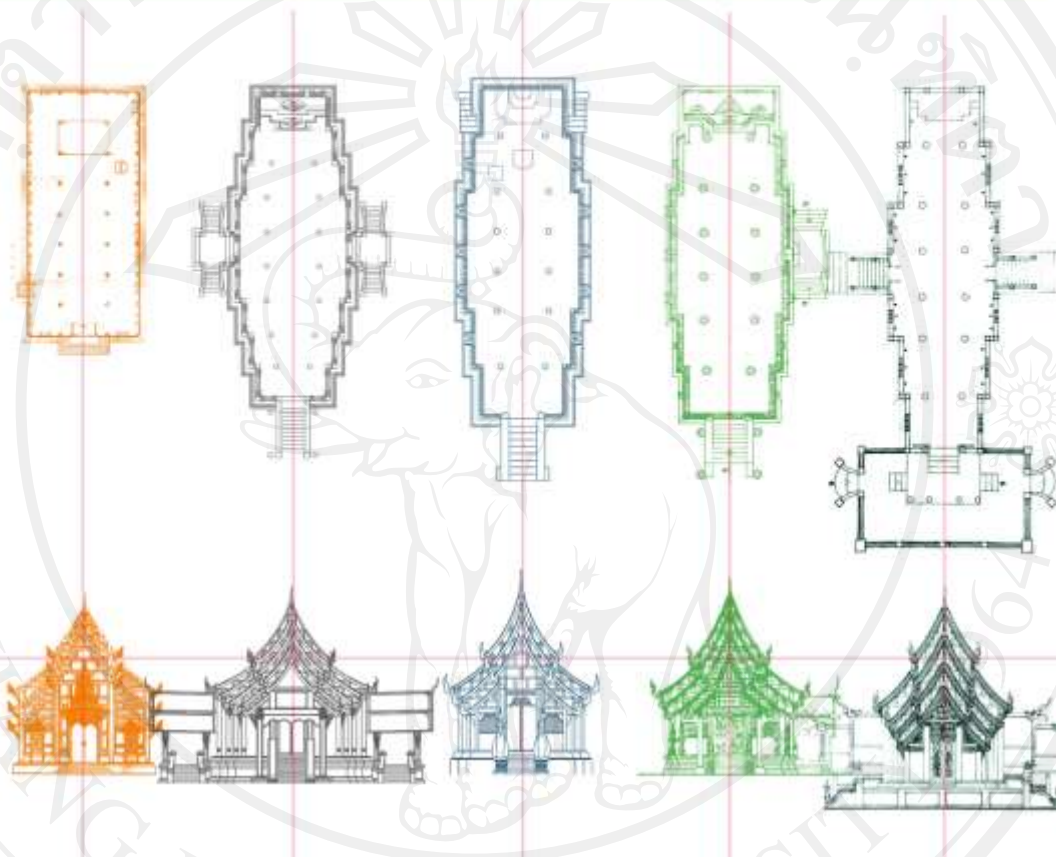
ภาพ 4-10 แสดงรายละเอียดการเปรียบเทียบรูปด้านหน้าและผังพื้นของวิหารล้านนา กลุ่มที่ 3 ประกอบด้วย วิหารวัดพันเตา วิหารวัดเกตุการาม วิหารวัดเสาหิน วิหารวัดบวรกรกหลวง และวิหารวัดท่าข้าม
