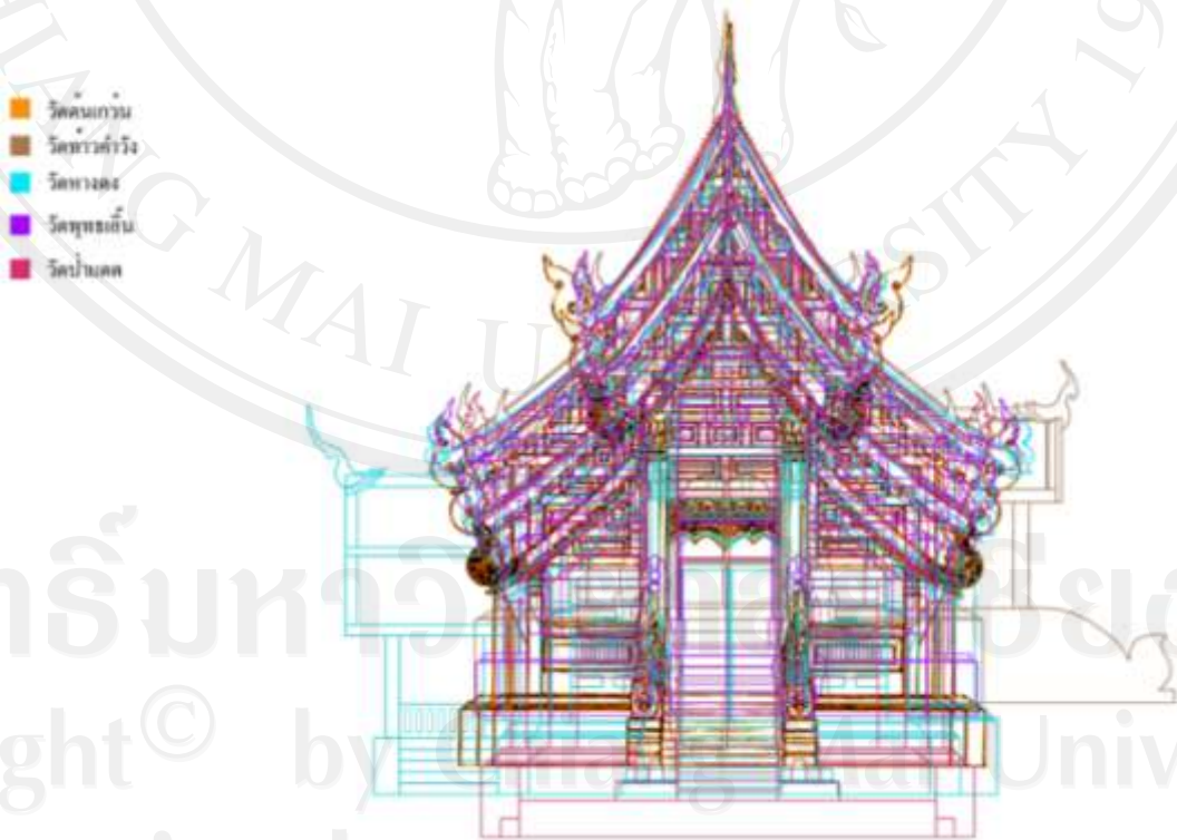
ภาพ 4-7 แสดงภาพเชิงซ้อนเปรียบเทียบรูปด้านหน้าของวิหารล้านนาในกลุ่มที่ 2 ประกอบด้วย วิหารวัดต้นแก้ว วิหารวัดท้าวคำวัง วิหารวัดหางดง วิหารวัดพุทธเอ็น และวิหารวัดป่าแดด
