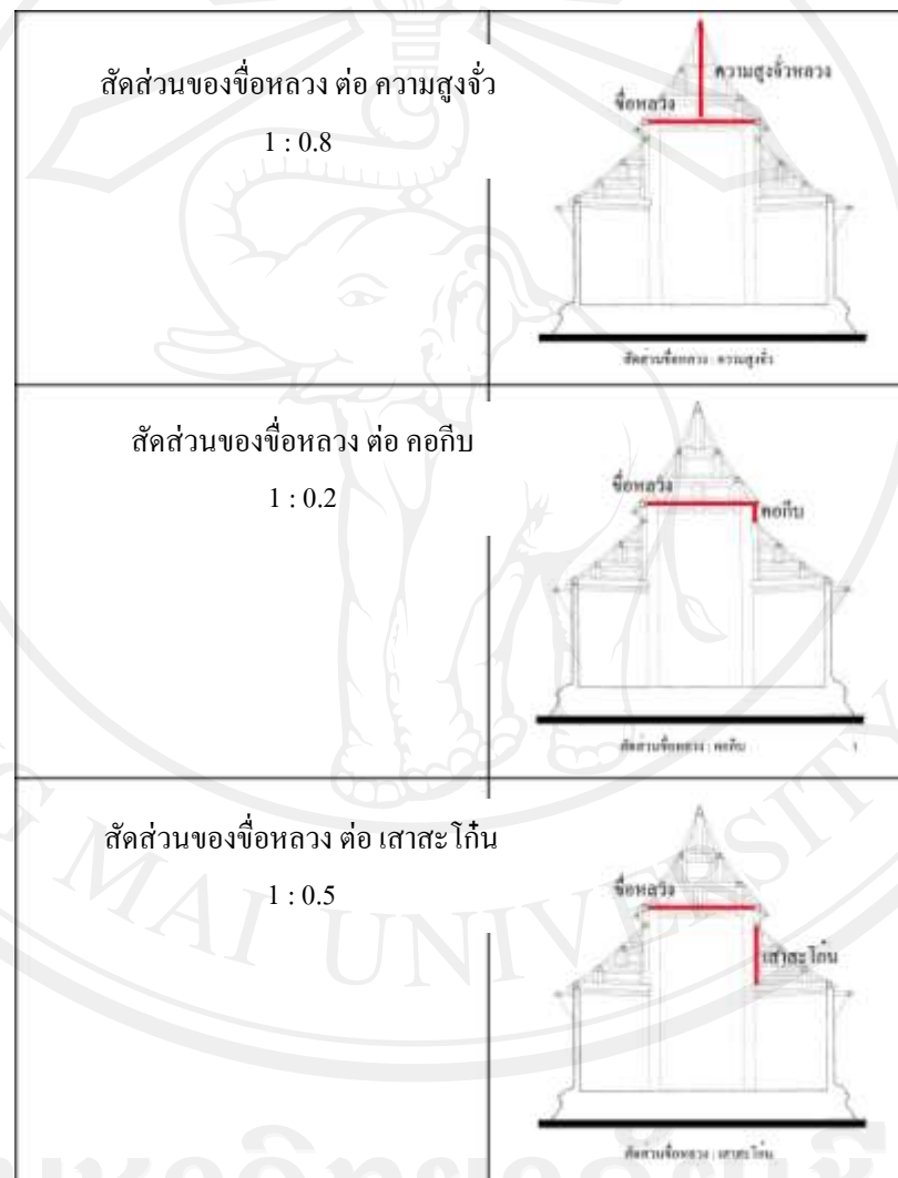
ภาพ 4-15 แสดงสัดส่วนวิหารล้านนาในจังหวัดเชียงใหม่
