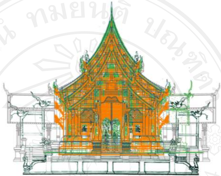
ภาพ 4-9 แสดงภาพเชิงซ้อนเปรียบเทียบรูปด้านหน้าของวิหารล้านนากลุ่มที่ 3 ประกอบด้วย วิหารวัดพันเตา วิหารวัดเกตการาม วิหารวัดเสนาหิน วิหารวัดบวรศรีพรหมหลวง และวิหารวัดท่าข้าม
