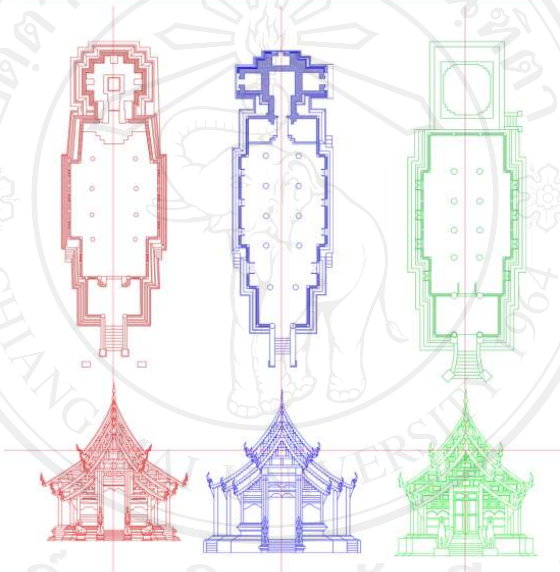
ภาพ 4-6 แสดงรายละเอียดการเปรียบเทียบรูปด้านหน้าและผังพื้นของวิหารล้านนากลุ่มที่ 1
