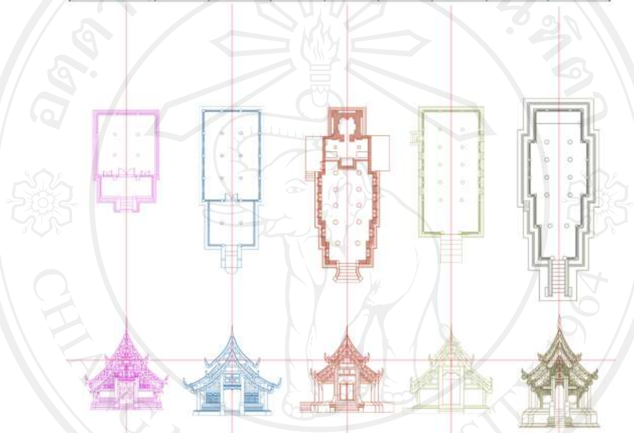
ภาพ 4-14 แสดงรายละเอียดการเปรียบเทียบรูปด้านหน้าและผังพื้นของวิหารล้านนากลุ่มที่ 4 ประกอบด้วยวิหารเล็กวัดบุพพาราม วิหารวัดป่าแดงหลวง วิหารวัดหัววัน วิหารวัดยางหลวง และ วิหารวัดวัดทุ่งฮ้อ
